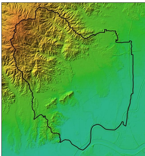
図 1-8 色別標高図
