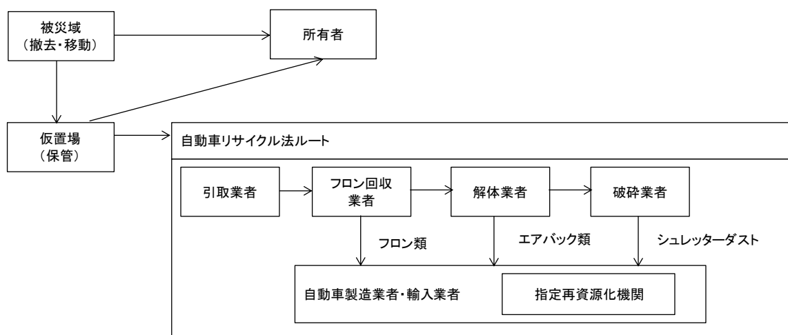
図 2-11 被災自動車の処理フロー
