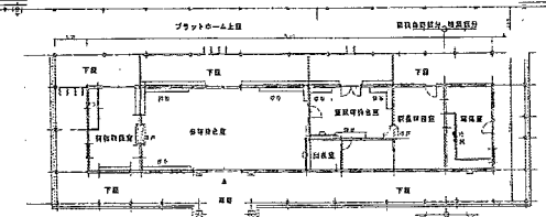
鳥栖駅本屋 第2期工事後の大正初期復原平面図
