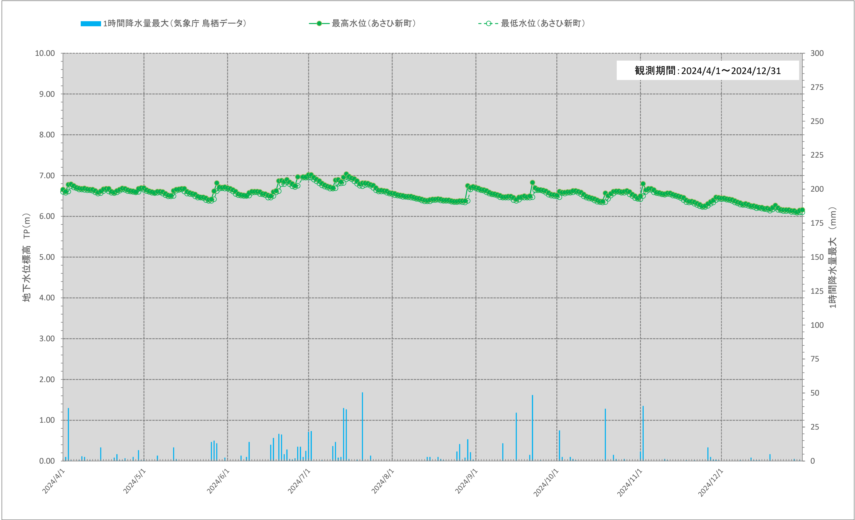
地下水位観測結果図(標高水位) 【あさひ新町】
