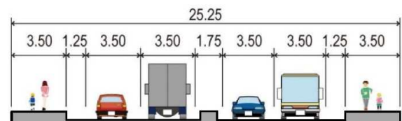
▲ 標準断面図
