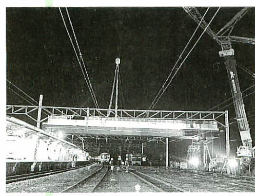
線路をまたぎ、橋脚上に設置される桁
