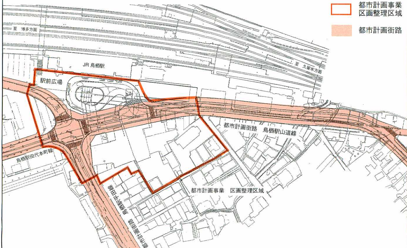
鳥栖駅西地区の道路及び区画整理事業計画図(案)
