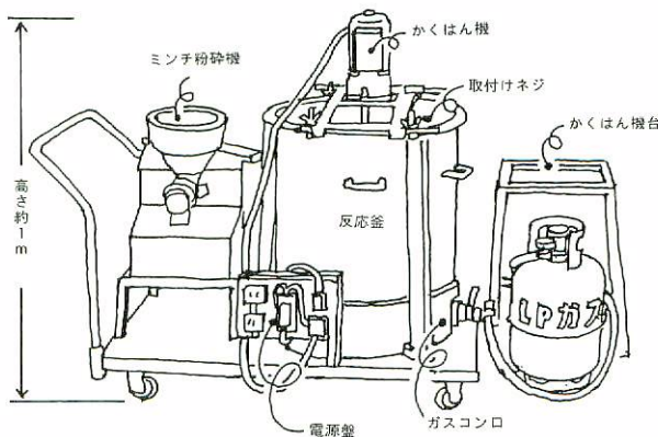
粉せっけんミニプラント
