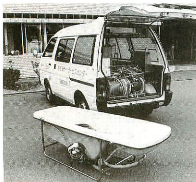
浴槽、ボイラーなどを備えた訪問入浴車
