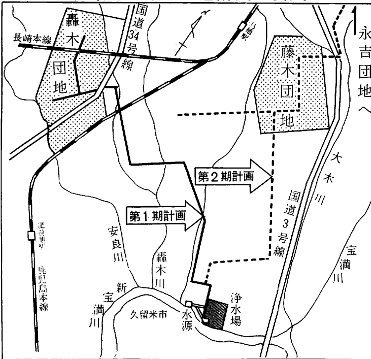
佐賀東部工業用水道計画概要図
