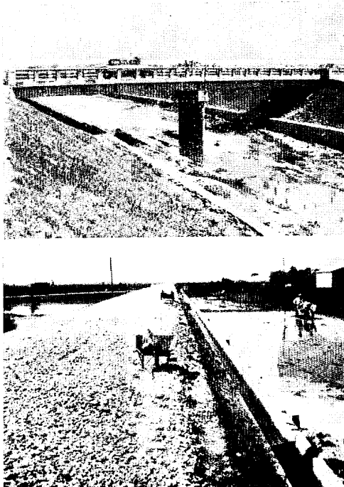
上 永久橋にかけられた日恵寺橋 中 農作業も便利になった永吉農道 下 改修された秋光川護岸工事と新設された井ぜき
